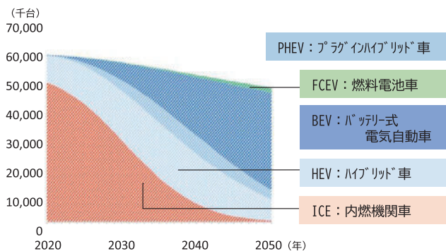
日本の乗用車保有構成： 電動化積極推進のシナリオ
