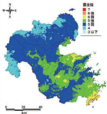
南海トラフ地震の震度分布（想定）
