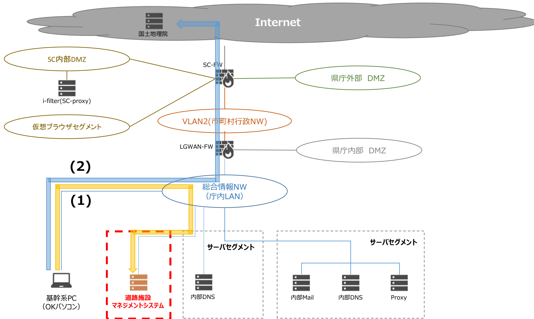
別紙②_ネットワーク構成図
