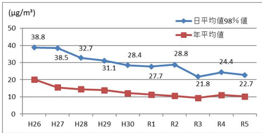
図 1-1-6(b) 微小粒子状物質に係る年平均値及び日平均値の経年変化(自動車排ガス測定局)
