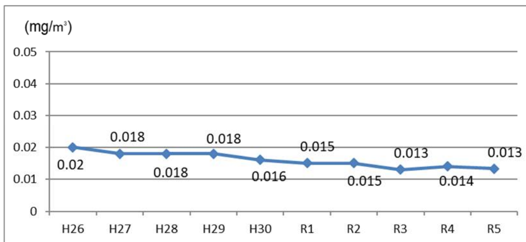
図 1-1-4(a) 浮遊粒子状物質に係る年平均値の経年変化(一般環境大気測定局)
