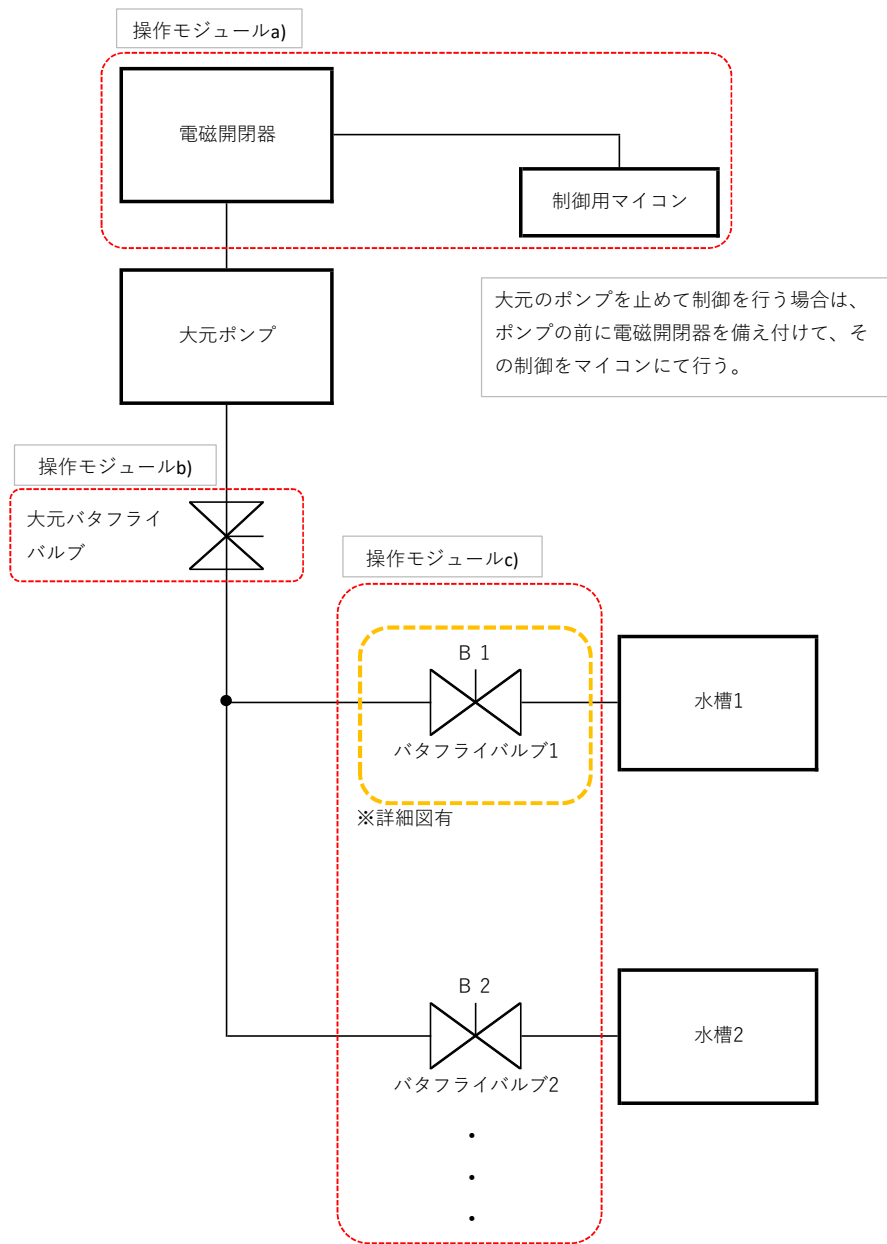
大分県水路制御系統図
