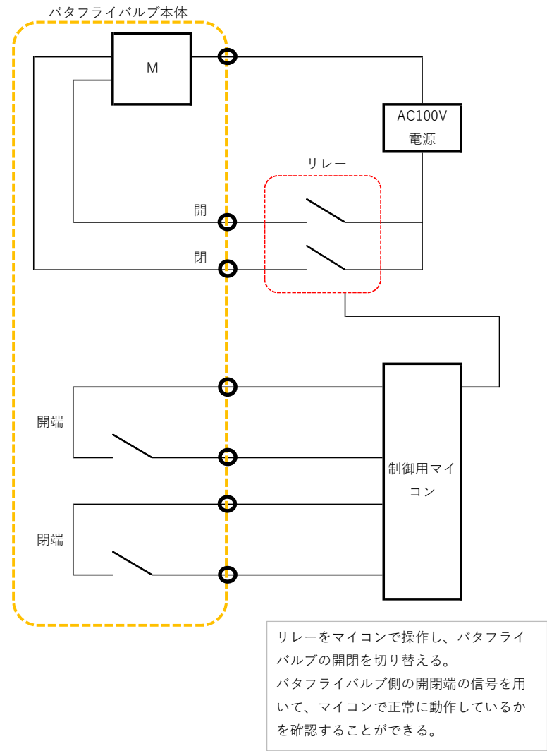
バタフライバルブ制御回路
