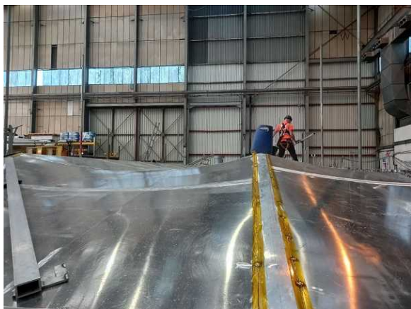
船底外板取付
