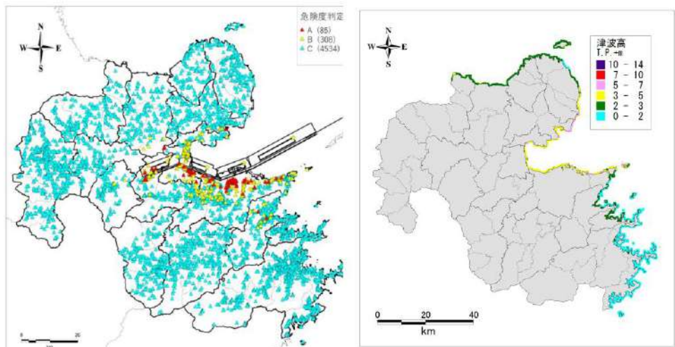
急傾斜地地震時危険度分布
