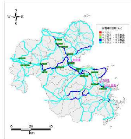
プレート内地震
