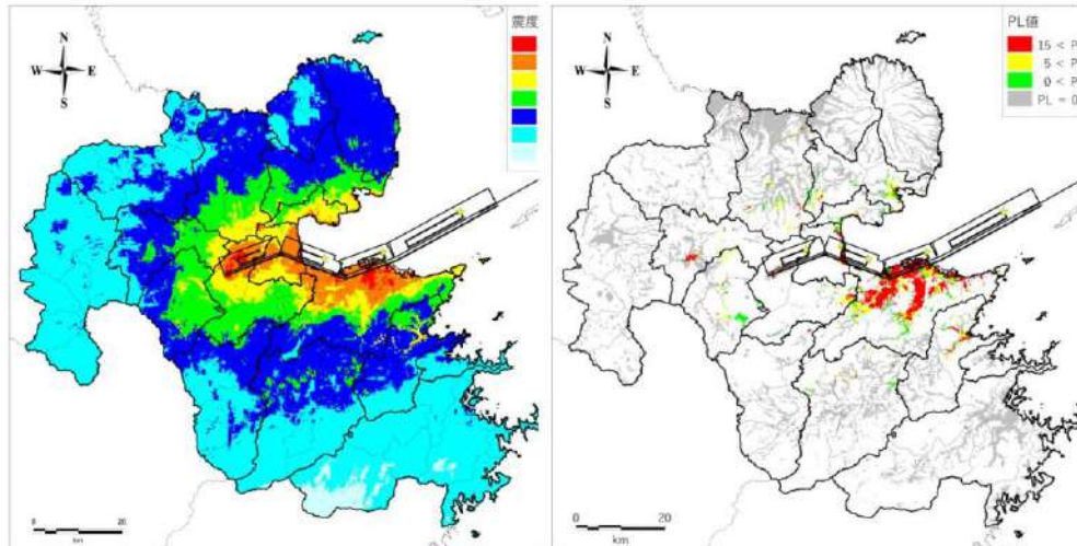
地表震度分布
