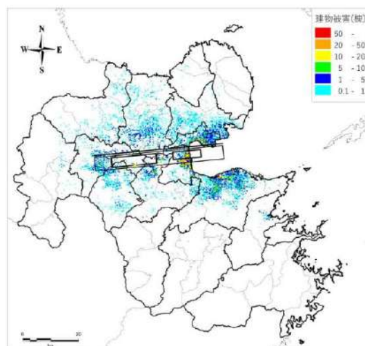
日出生断層帯による地震
