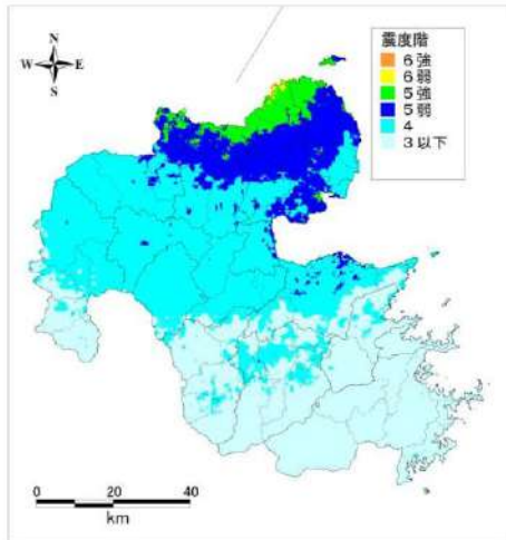
地表震度分布図
