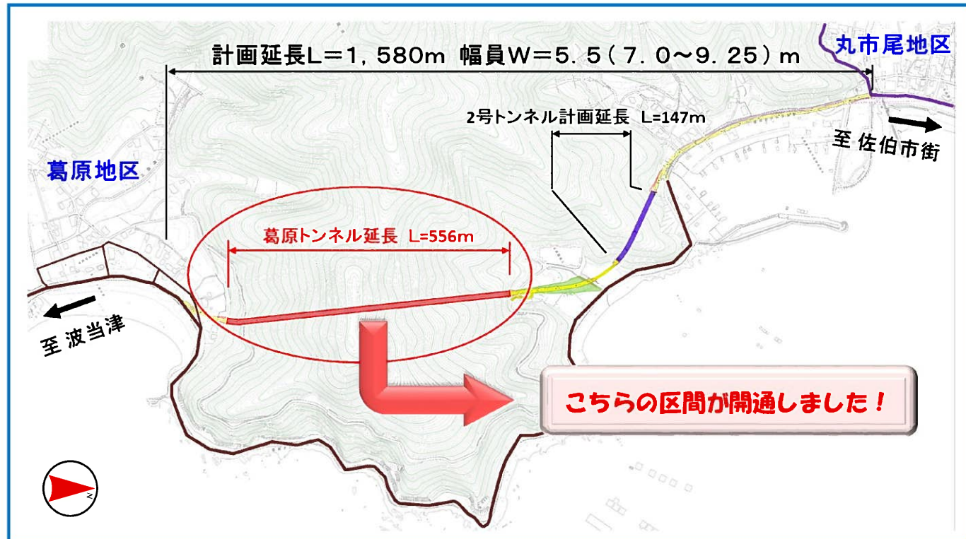
<<古江丸市尾線(葛原～丸市尾工区)計画図>>
