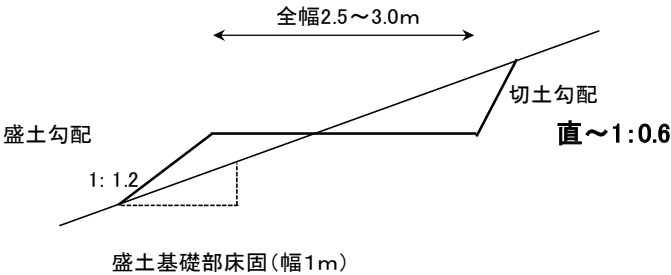
土工標準図
