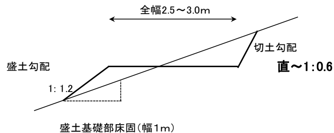
土工標準図
