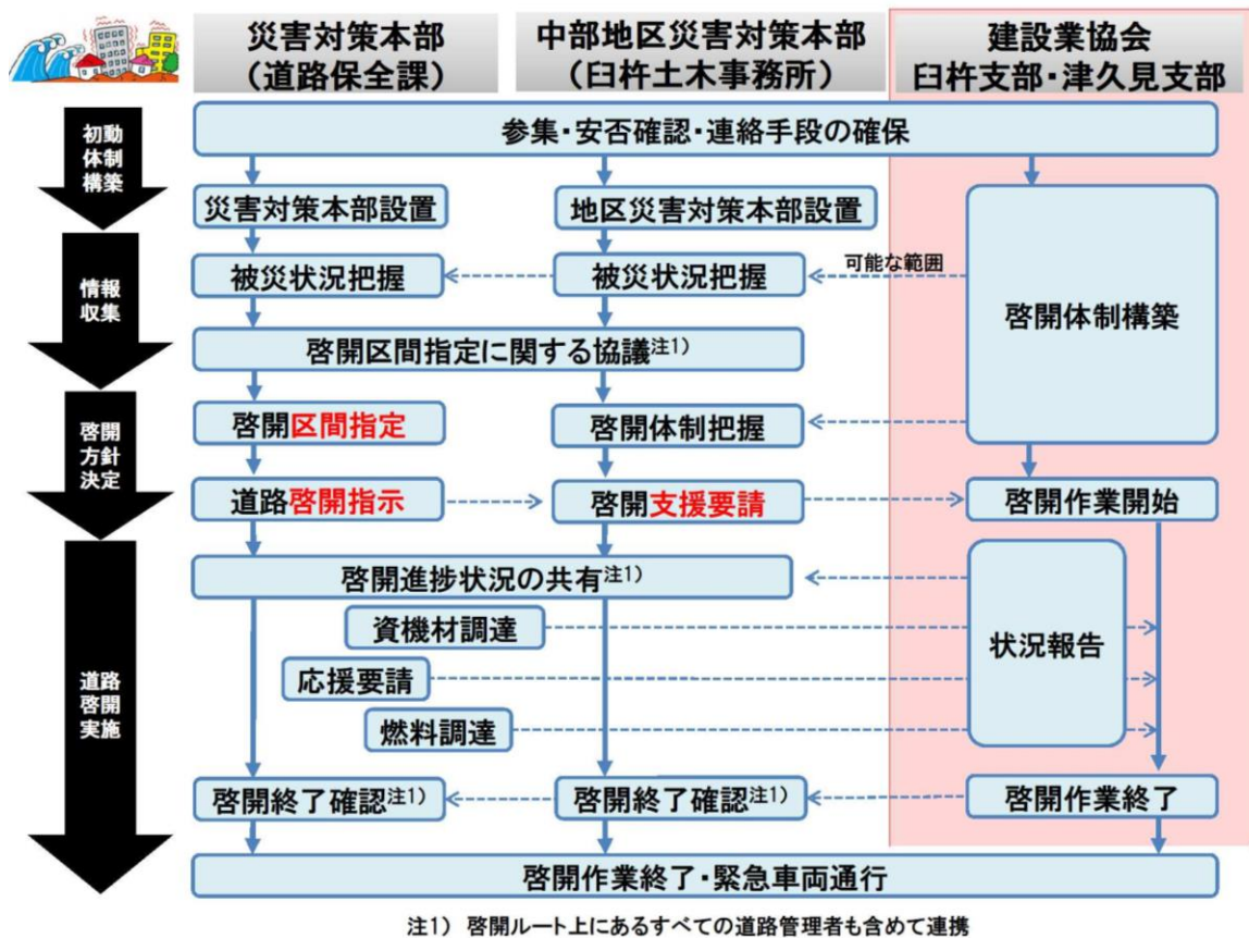
図6 建設業協会 臼杵支部・津久見支部における道路啓開手順
