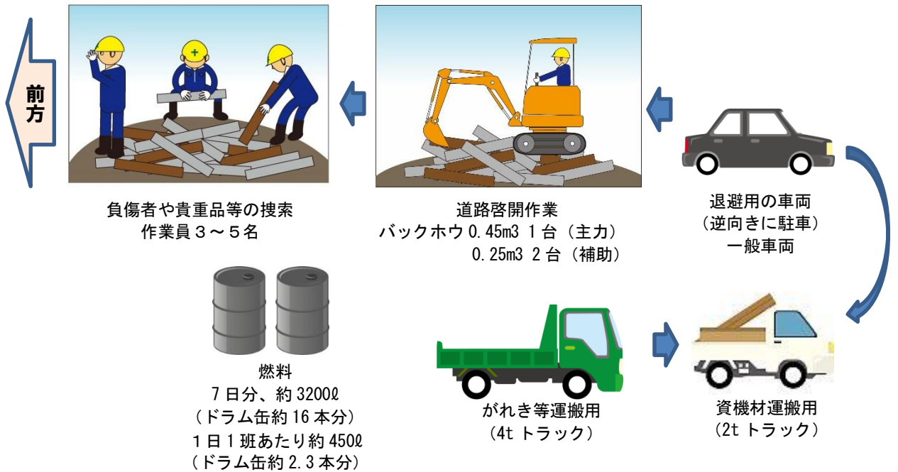
図9 標準的な班編成（作業員8～10名）
