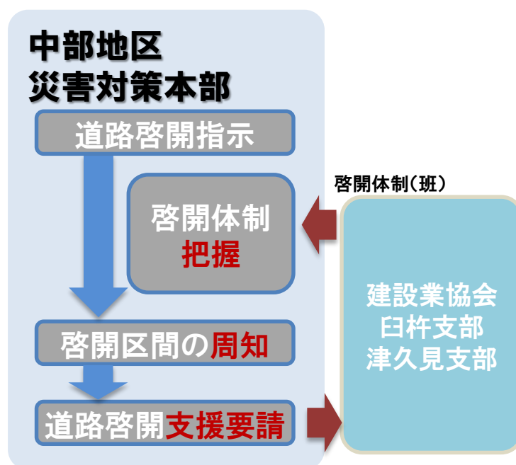
図 4 地区災害対策本部における道路啓開作業の開始手順
