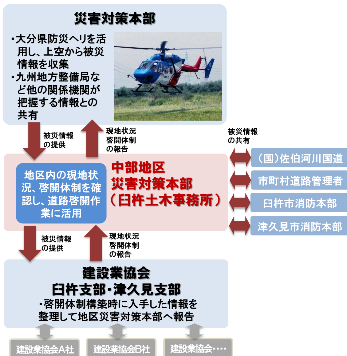
図3 被災情報の収集・整理体制
