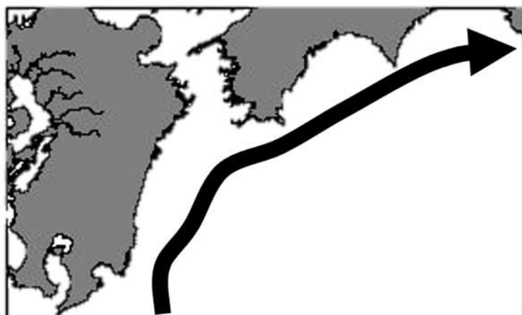
黒潮流路図
