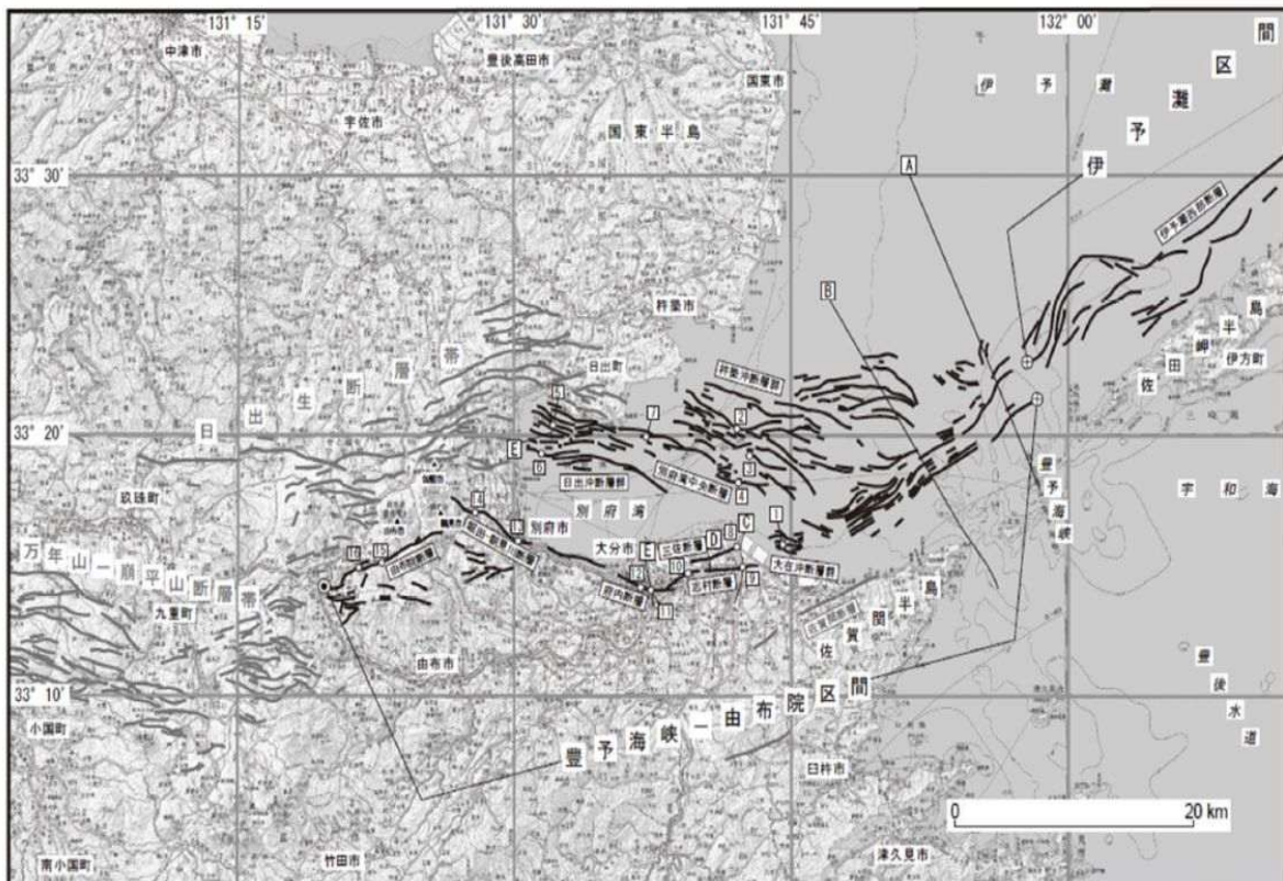
中央構造線断層帯の活断層位置と主な調査地点
