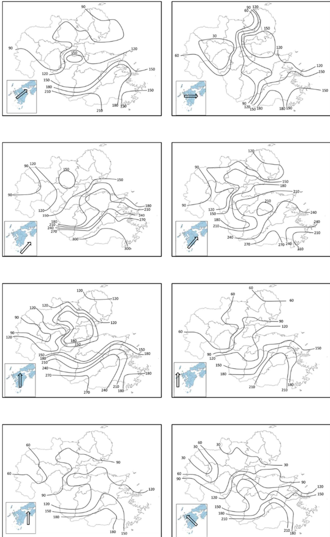
台風の経路と大分県の雨量分布
