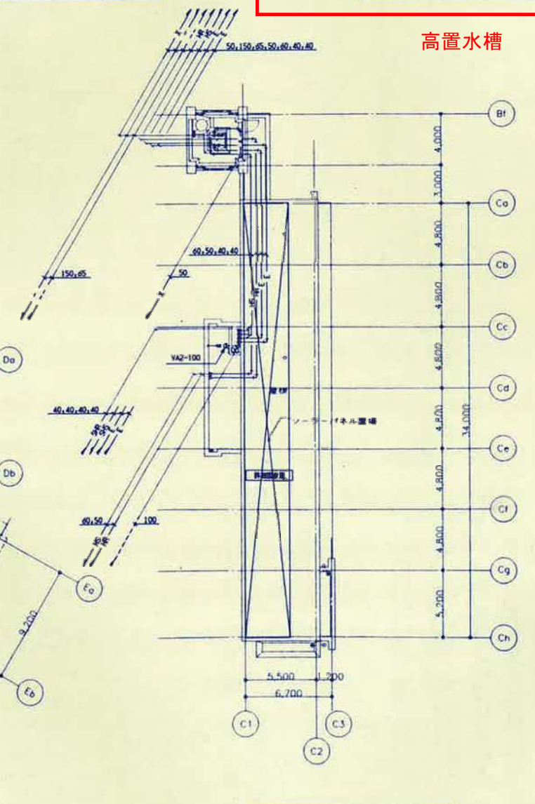
屋根平面図 S:1/200
