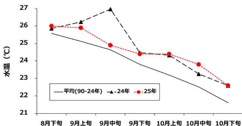
定地水温(表面:°C) [佐伯湾奥]
