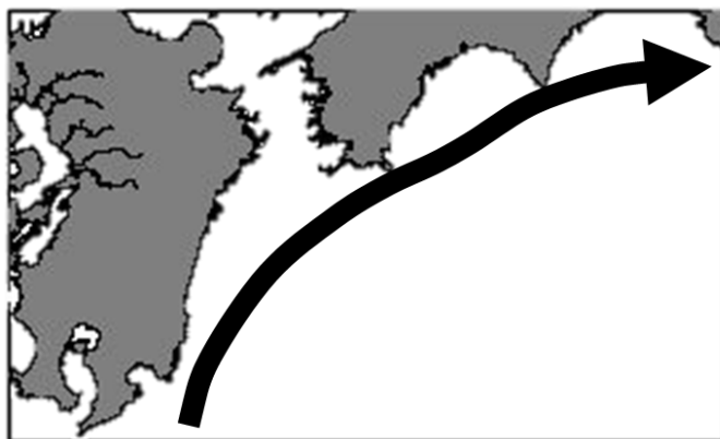
黒潮流路図
