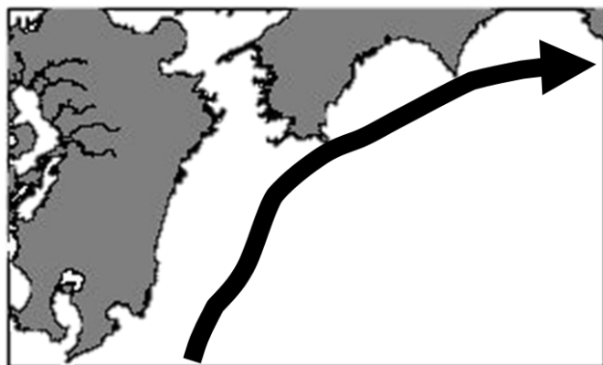
黒潮流路図
