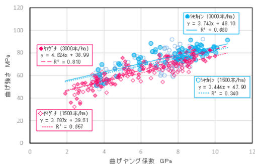
図-1 植栽本数別、品種別の曲げヤング係数と曲げ強さの比較
