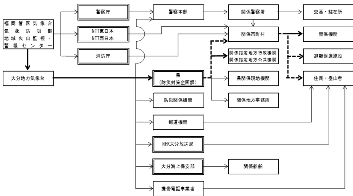
図 5-1 噴火警報・予報等の情報伝達系統図
