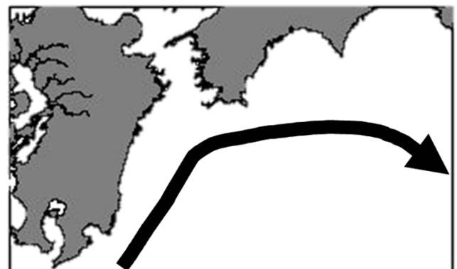
黒潮流路図
