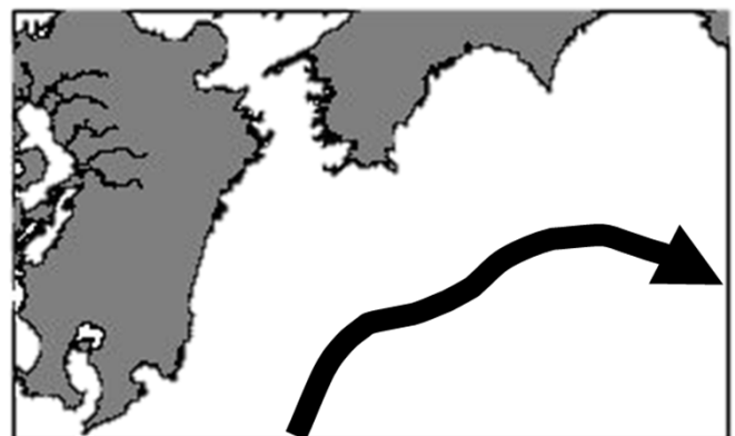
黒潮流路図
