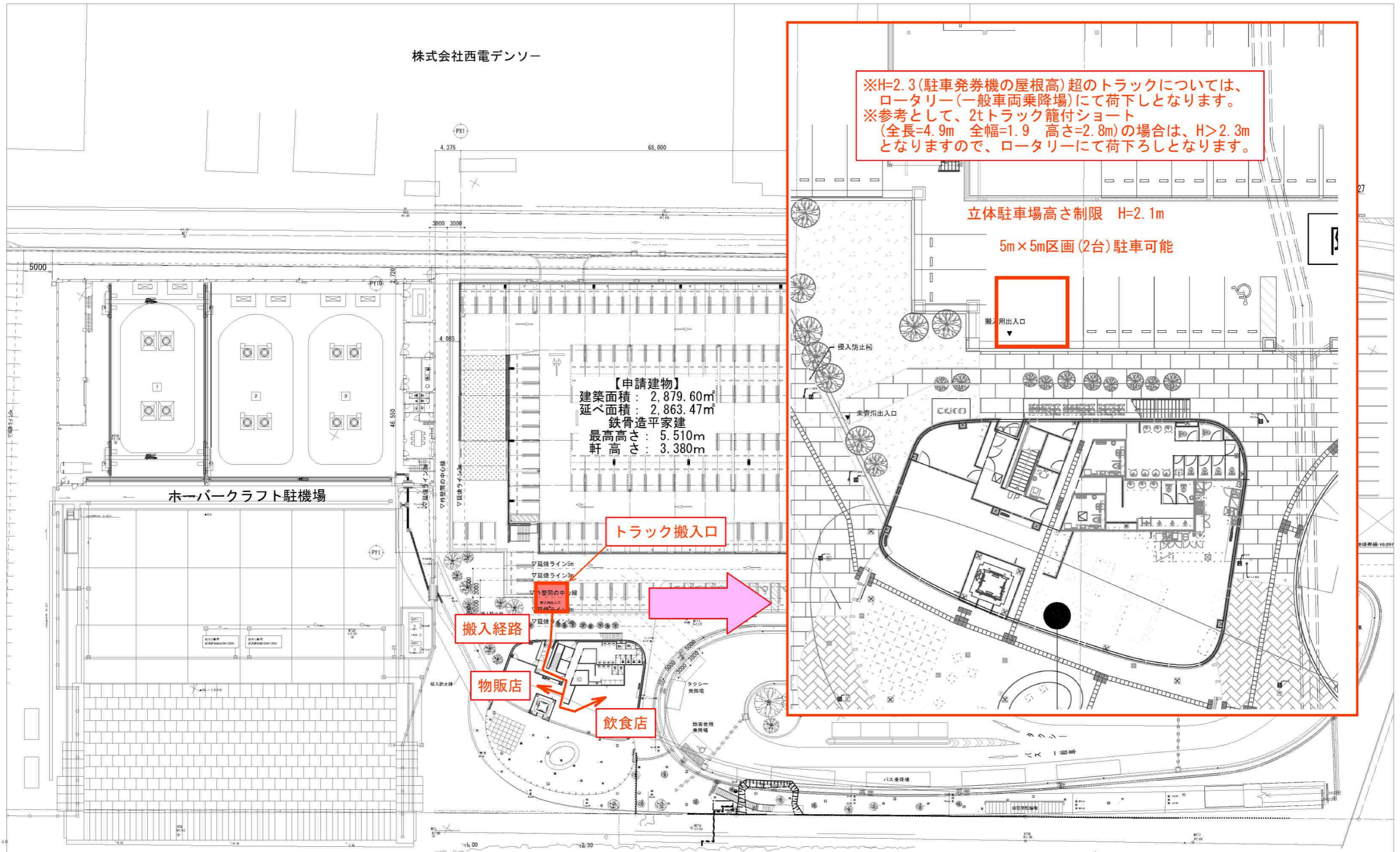
配置図 1/300 ・駐車場GL±0(2.40)=KBM2(2.627)-0.227
