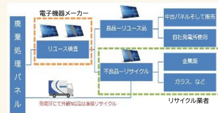
全国初となる自社開発装置による太陽光パネルのリユース&リサイクル
