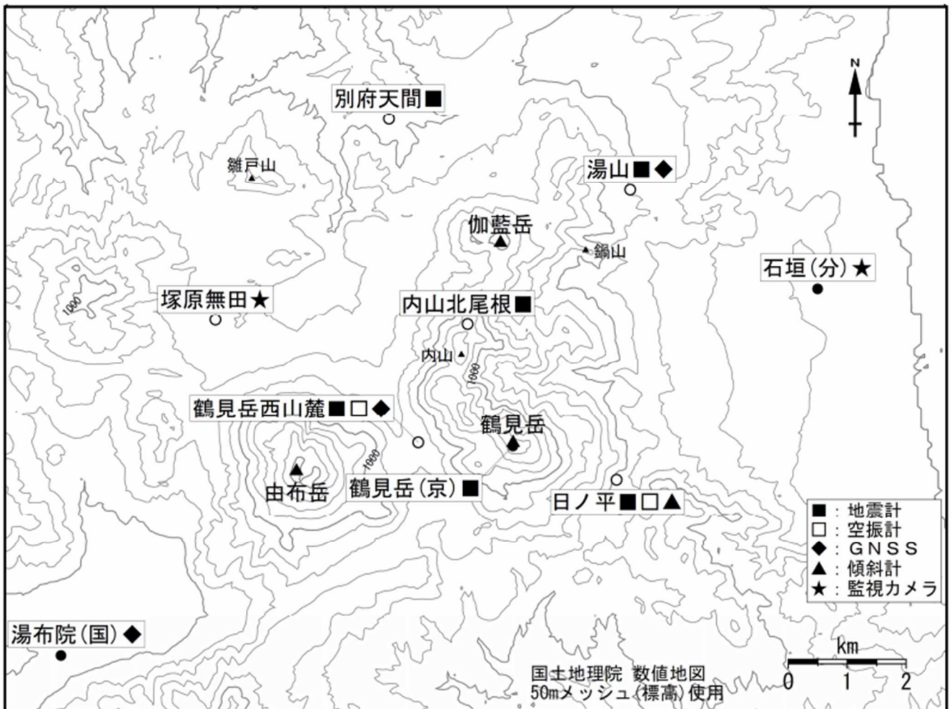
図 2-5 鶴見岳・伽藍岳観測点配置図（気象庁ホームページより）
