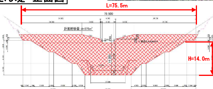
えん堤 正面図
