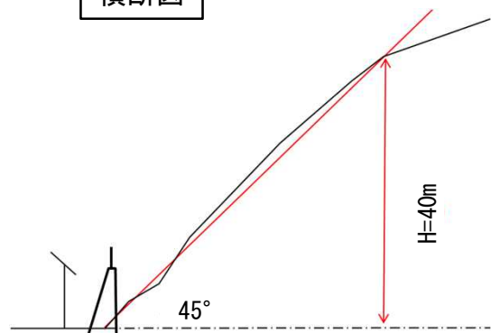
横断面図
