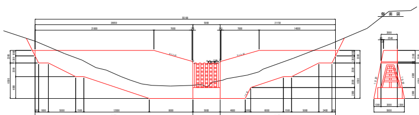
透過型堰堤正面図
