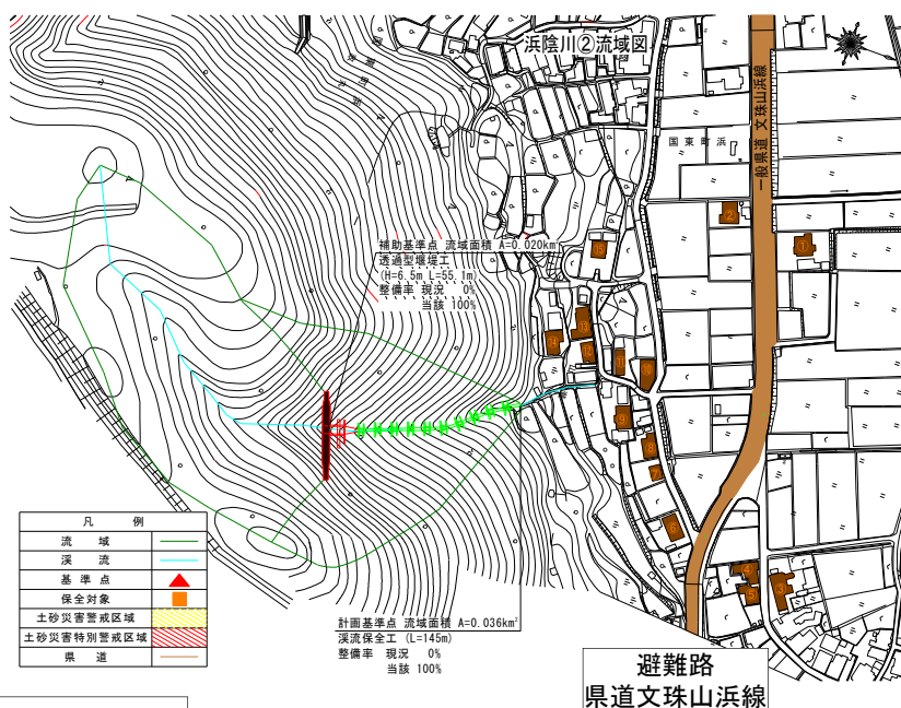
施工計画図
