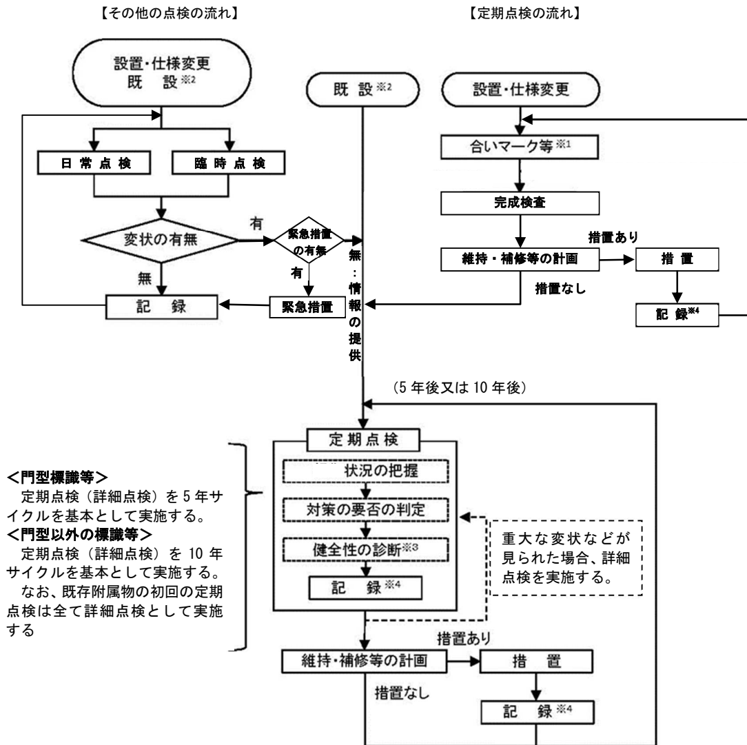
図 5-1点検の流れ
