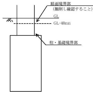
図-解 8-2 路面境界部の定義
