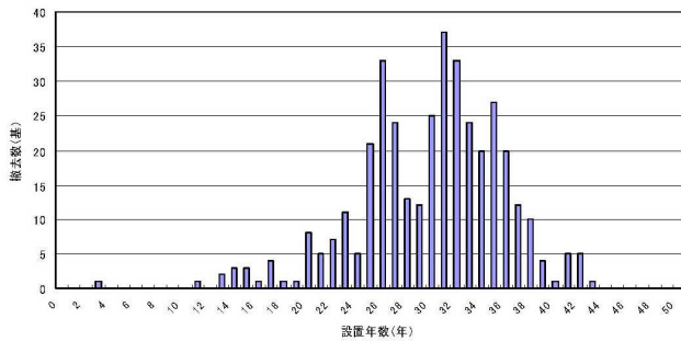
(a) 道路照明
