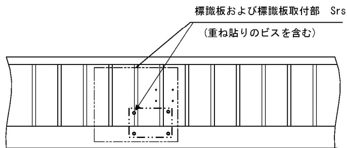
図-解 8-11 主な点検箇所 (添架式)
