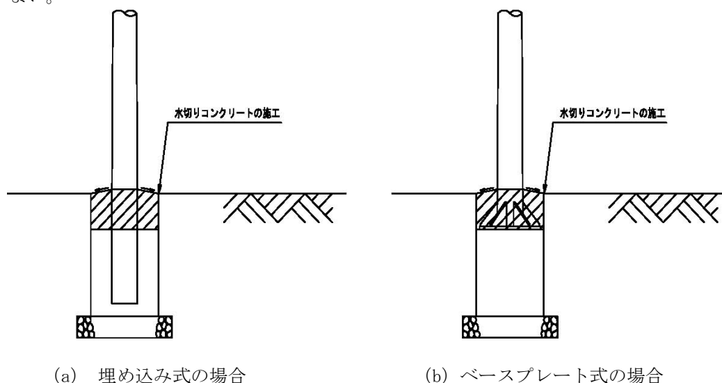
図-解 12-1 水切りコンクリートの施工イメージ
