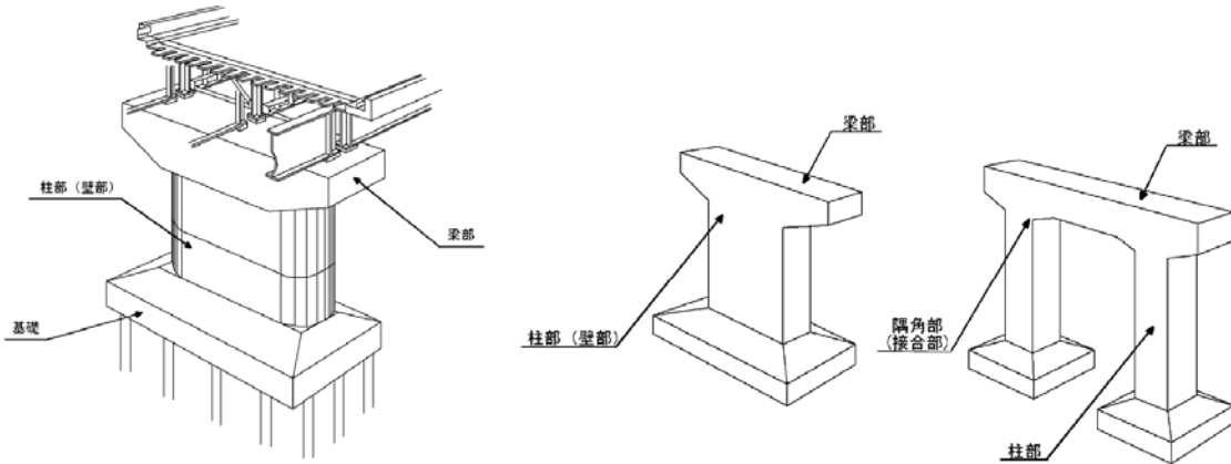
橋脚
