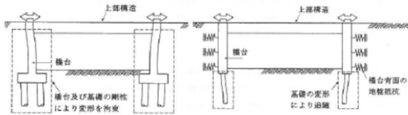
橋台部ジョイントレス構造
